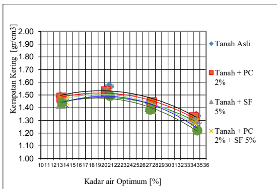
Gambar 4. Grafik Perbandingan Campuran terhadap Pematatan Tanah
